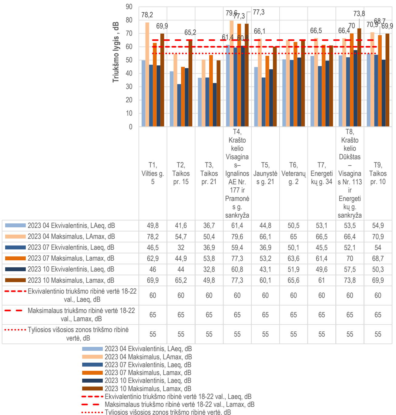
4.3 pav. Ekvivalentiniai ir maksimalūs triukšmo lygiai vakaro metu (18-22 val.)
