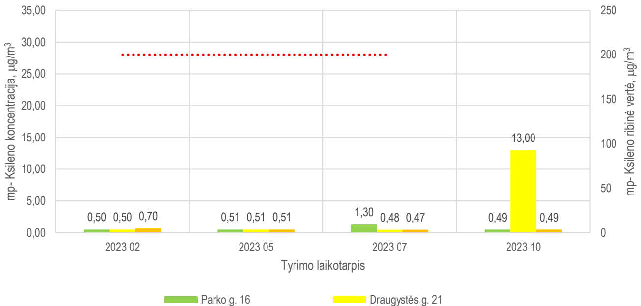
5.10 pav. mp- Ksileno koncentracija aplinkos ore
