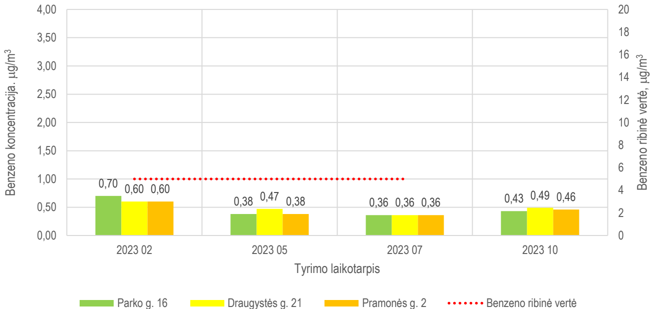
5.6 pav. Benzeno koncentracija aplinkos ore
